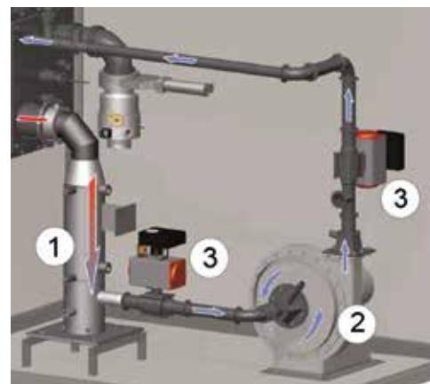
Rappresentazione schematica del raffreddamento rapido a gas
